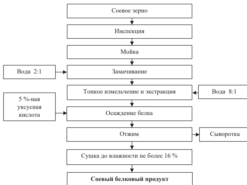
Рисунок 1. Технологическая схема производства соевого белкового продукта
